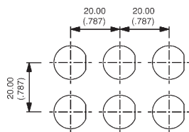
Einbauraster
