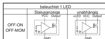
Schaltschema
