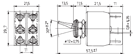
Serie 600NH 2-polig mit isoliertem Hebel
