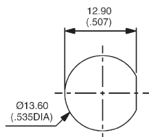
Einbaudurchmesser
