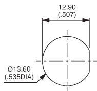
Einbaudurchmesser
